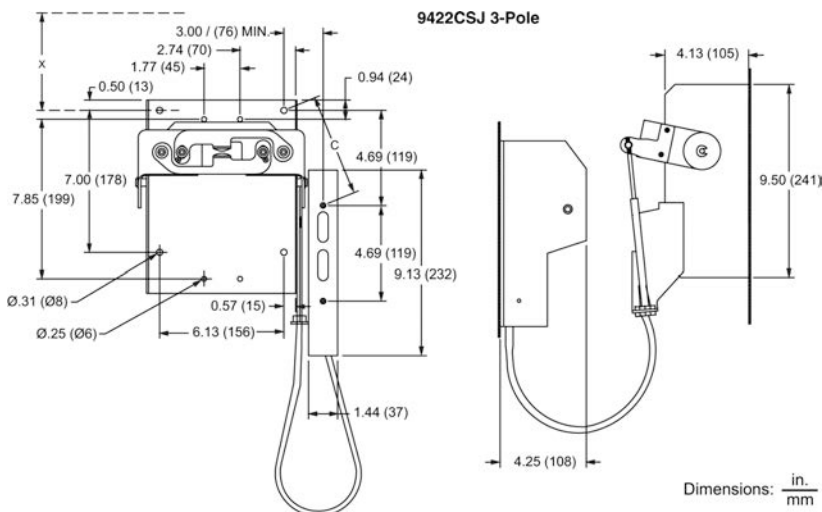
9422CSJ 3-Pole
