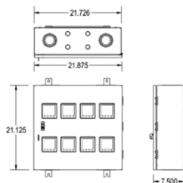
8 meter configuration
