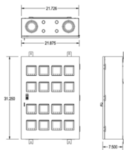
16 meter configuration
