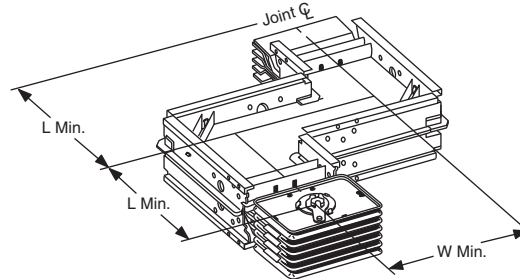
Flatwise: Catalog Number Suffix–OF
